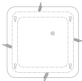
Защелки в положении «Открыто»
